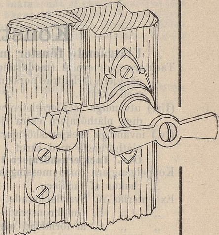
Stängselvred till enbågiga fönster. Half storlek.
