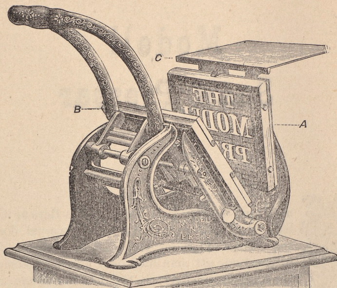
Fig. 1. Modell Snällpress No. 3.
