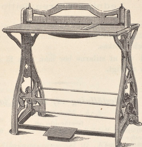
Fig. 15 Perforeringsmaskin Pris Kr. 350.
