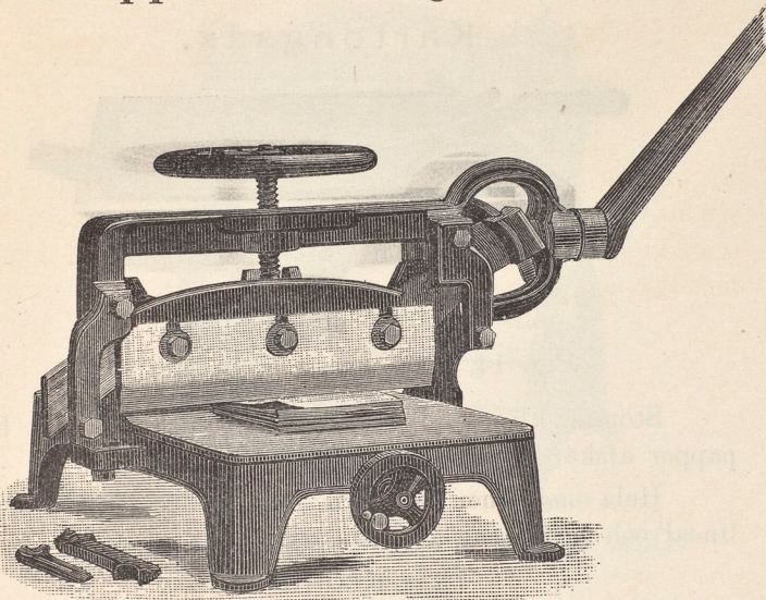
Fig. 13. Pappersskärningsmaskin N:o 1. Skärlängd 12 v. t.
