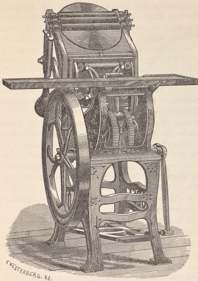
Fig. 4. Sjelffärgande Modell-Snällpress Nr 5. att drifvas med tramp eller rem.
