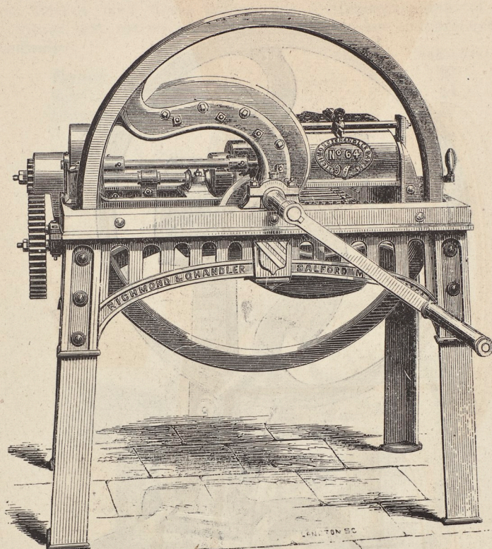
Patent-Hackelsemaskin N:o 64.
