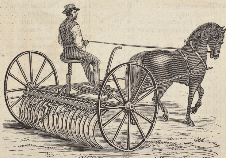
Amerikansk hästräfsa.
