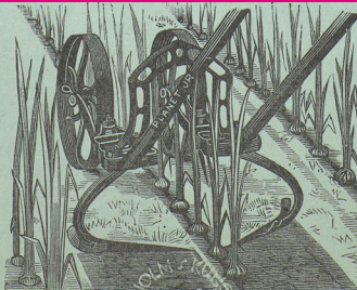
"Planet j:r". Tvåhjulig hacka.
