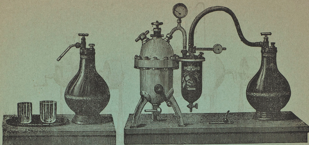
Hushällsapparat C.
