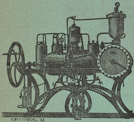
Sodavattenapparat B.
