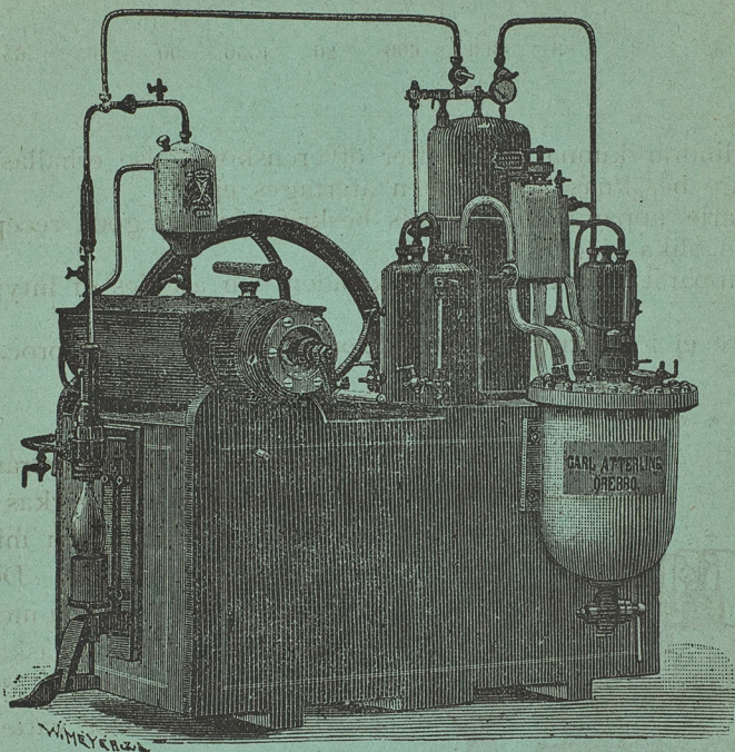
Sodavattenapparat A.
