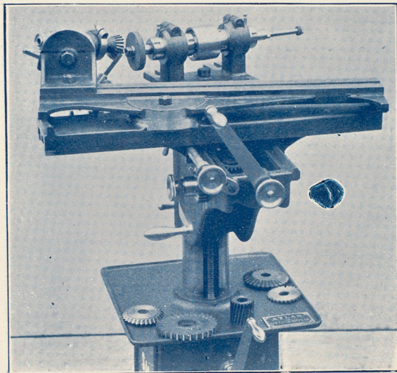
Skärpning af frästrissor.
