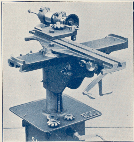
Skärpning af frästrissor.
