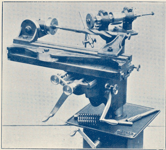
Skränkning af spiralborrar.
