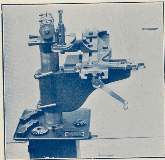
Fasonsliپning efter ledare.
