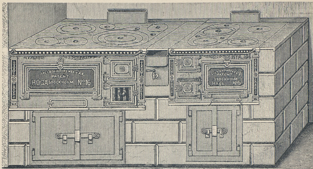
N:is 16 och 6 med en kopparcistern, 2 varmugnar och mellanplåtar. 1,850 mm. lång, 690 mm. bred, 765 mm. hög.
