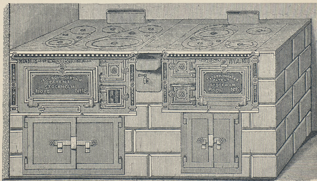
N:is 18 och 6 med en kopparcistern, 2 varmugnar och mellanplåtar. 1,710 mm. lång, 685 mm. bred, 765 mm. hög.
