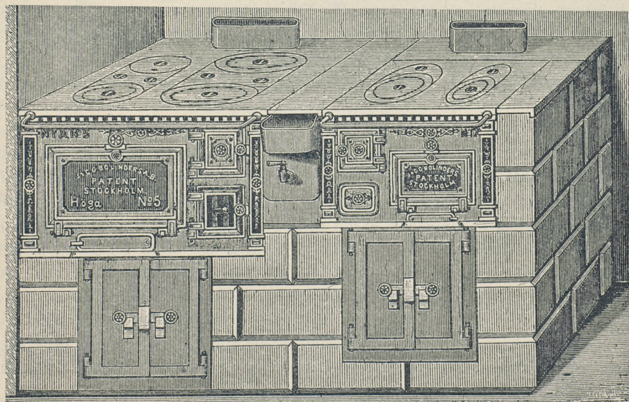
N:is 5 och 17 med en kopparcistern, 2 varmuvar och mellanplåtar. 1,510 mm. lång, 670 mm. bred, 765 mm. hög.
