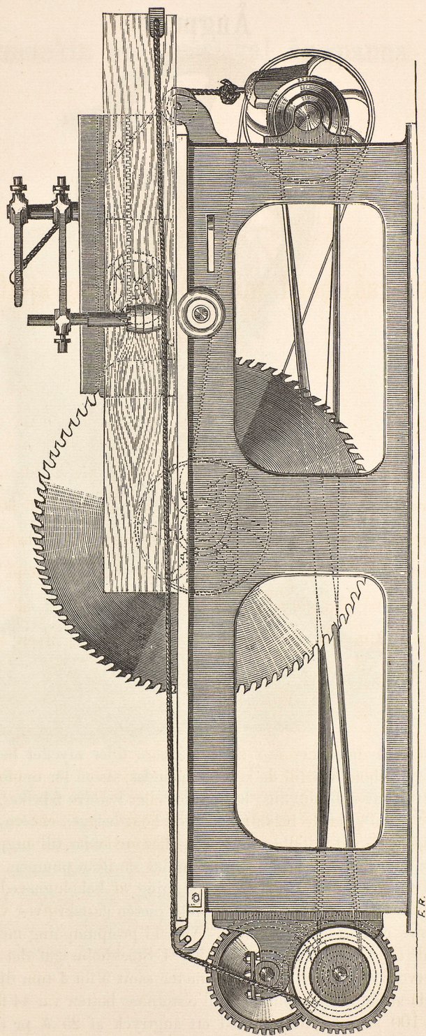
Cirkulärsågbord med föränderlig sjelfverkande matning.
