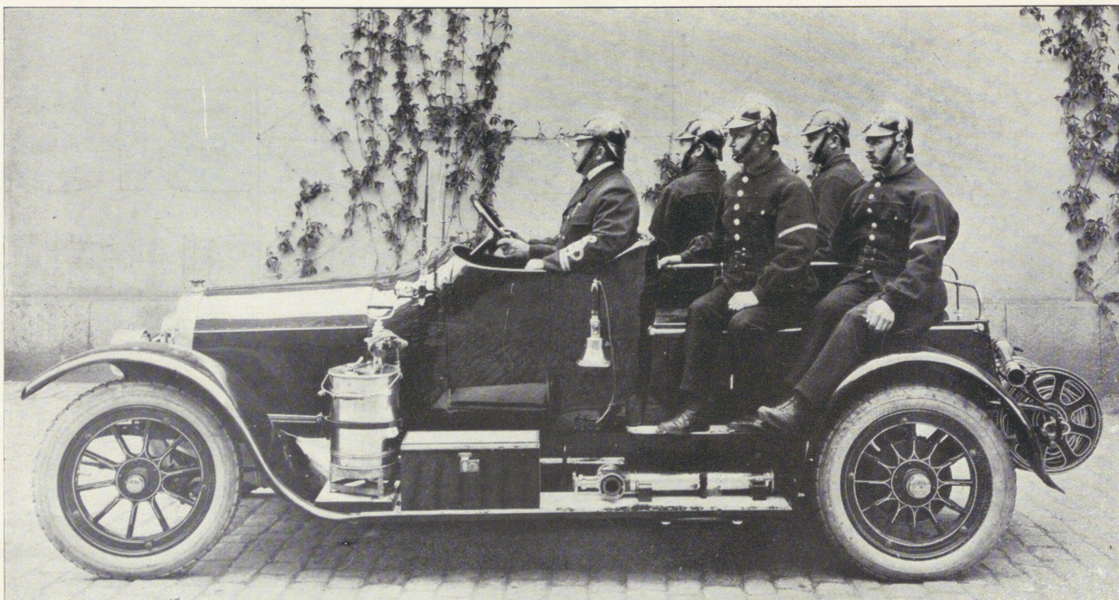
En af Stockholms Brandkårs 30 Hkr. SCANIA-VABIS MANSKAPS- och REDSKAPSAUTOMOBILER; går som första vagn vid utryckning; hastighet 70 km. pr tim.
