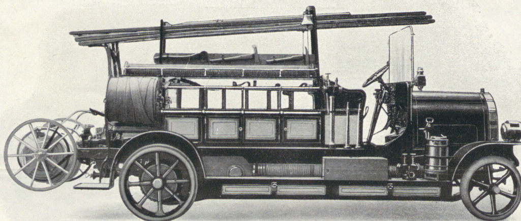
60 Hkr. 1500 minutilters SCANIA-VABIS AUTOMOBILSPRUTA med R. A. G.-pump.
