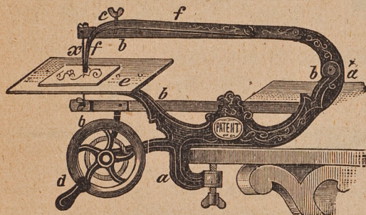
* Hand-Löfsågningsmaskin N:o 1. Sågvidd 35 centimeter. Kan äfven drifvas med tramp. Maskinen fastskrufvas å vanligt bord. Pris med ett dussin sågblad och skrufmejsel Kr. 10.
