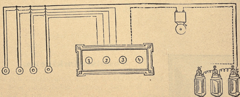
Schema för uppsättning af ringledning i samband med nummertafel.
