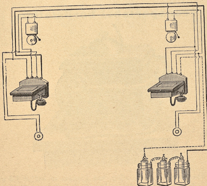
Uppsättningsschema för Mikrotelefon.
