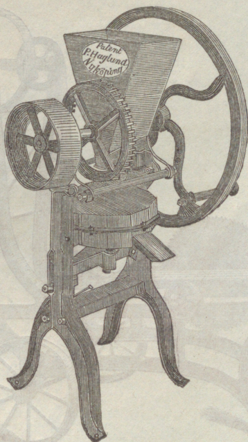
Fig. 41. Gröppqvarn, af P. Haglunds patent.
