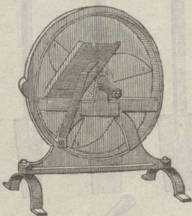
Fig. 40. Bön- och Gurkskärare.
