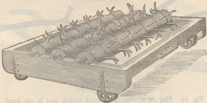
Fig. 10. Rullharf, med 3:ne axlar af träd, i hvilka smidda knifvar och pinnar äro fästade, samt med 4 transporthjul.
