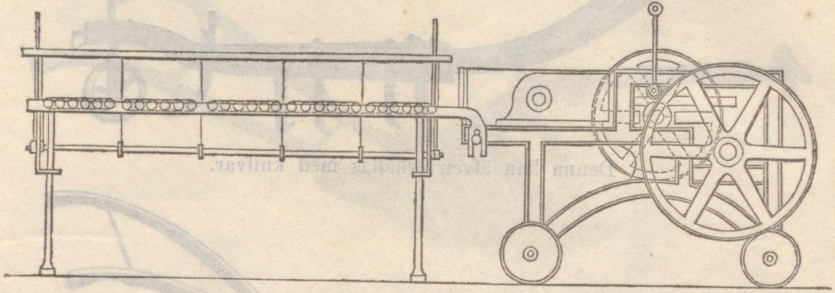
Fig. 29. Tegelrörsmachin, efter J. Whiteheads i Preston modell, förbättrad vid Näfveqvarn.
