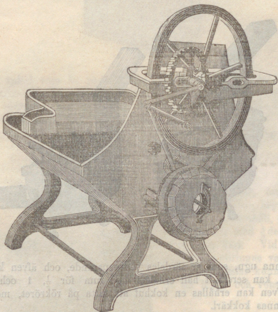
Fig. 28. Smedässja, med fläkt och härdho, helt och hållet af jern.
