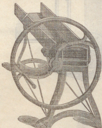
Fig. 3. Hackelsemachin.
