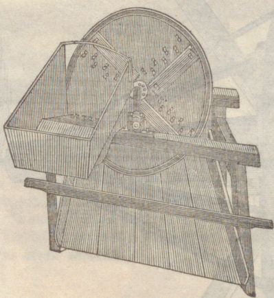
Fig. 4. Rotskärningsmachin.
