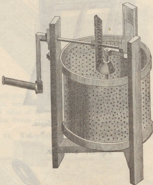
Fig. 38. Potatis-skalare.
