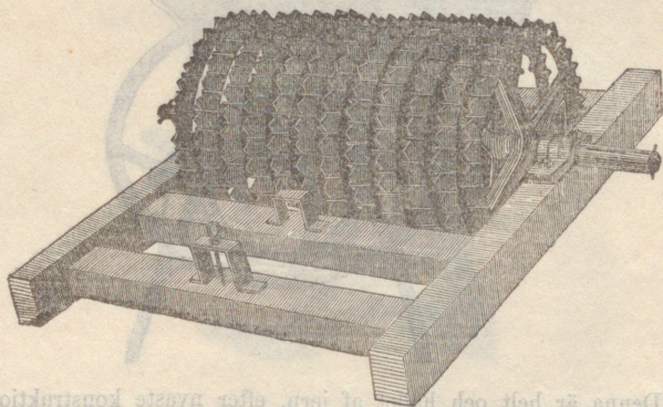
Fig. 8. Vält, efter Crosskils modell.
