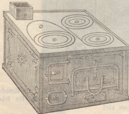
Fig. 33. Kokspisel № 7. Lika med Bolinders № 6.
