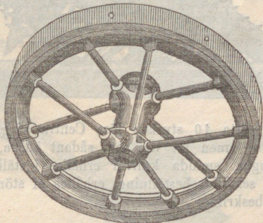
Fig. 7. Vagnshjul, med ekrar, skenring och bössa af smidt jern samt naf och lötring af gjutjern.
