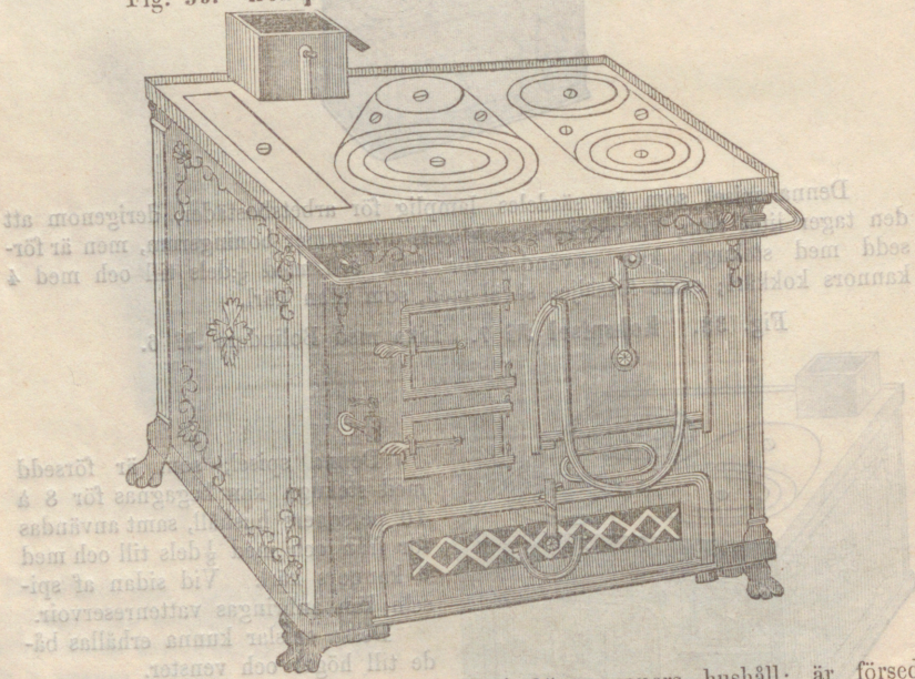
Fig. 35. Kokspisel № 9. Lika med Bolinders № 3.
