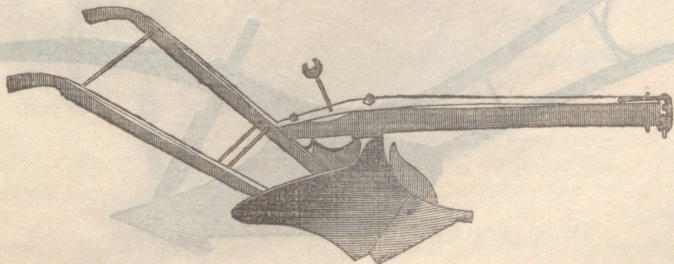
Fig. 18. Plog № 7. Lika med plogen № 4, men med smidd bill och rist.
