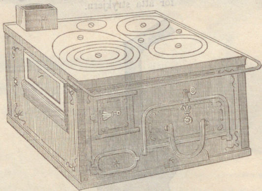
Fig. 34. Kokspisel № 8. Lika med Bolinders № 5.
