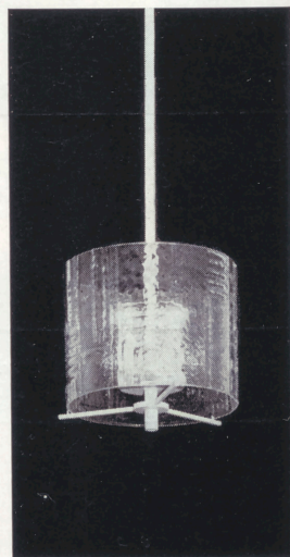
12678 Lackerad metall Klart glas Höjd 800 \phi 350 3×60 W
