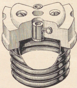
No. 7100. Патронъ Эдисона съ коробочнымъ контактомъ безъ выключателя. Изъ латуни вытравена.
