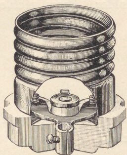
No. 7100. Douille Edison sans clé avec contact à boîte. Laiton déroché.
