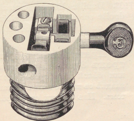
Но. 7110. Патронъ Эдисона съ выключателемъ съ коробочнымъ контактомъ. Изъ латуни отполиров.
