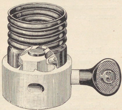
No. 7110. Douille Edison à clé avec contact à boîte. Laiton poli.
