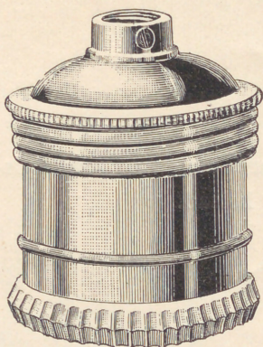
No. 7100. Edisonlamphållare utan vred med hyls-kontakt. Mässing betsad.
