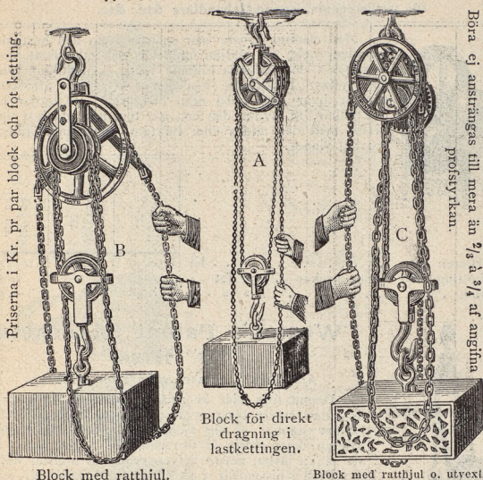
Block med rattghjul.
