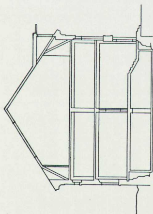
SEKTION A-A
