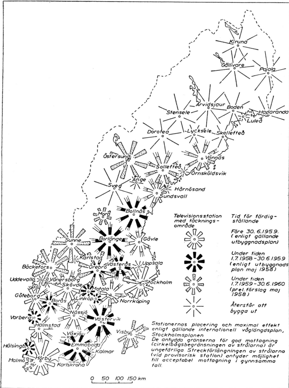
Fig. 1. Televisionssändare enligt kommunikationsdepartementets utbyggnadsplan.
