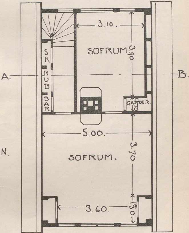
PLAN AF VINDSVÅNING.
