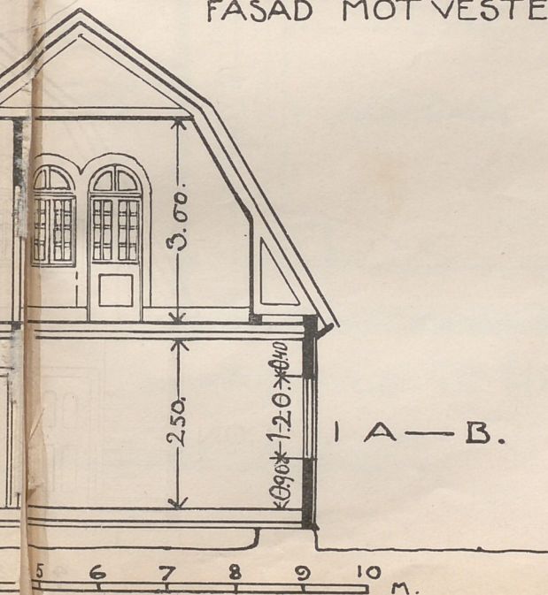
FASAD MOT VESTER.
