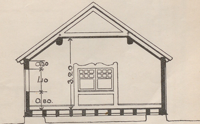
SEKTION I A - B.
