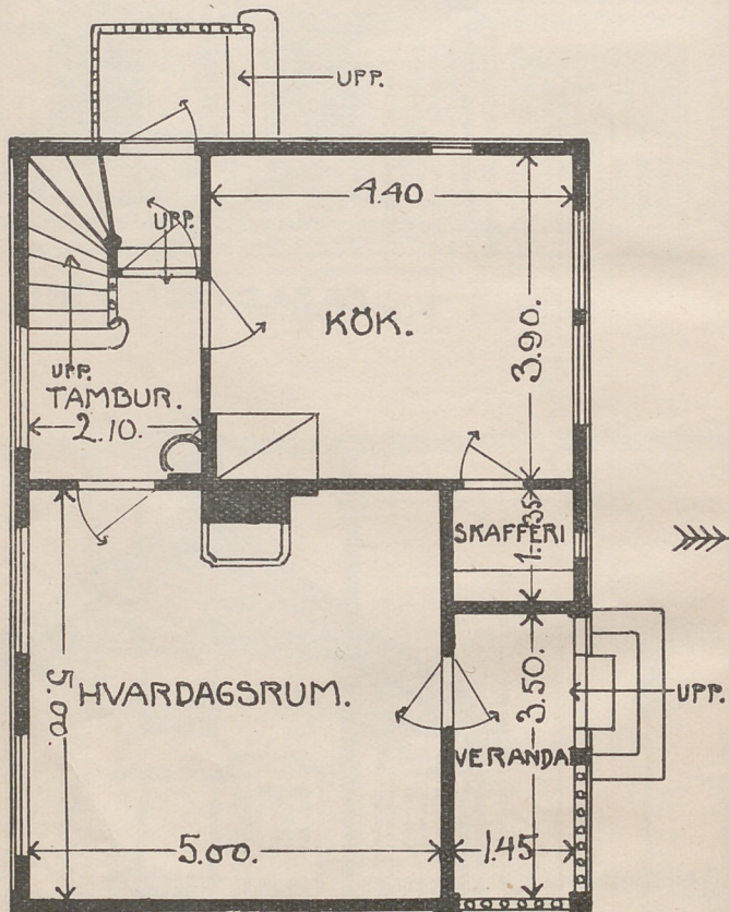
PLAN AF BOTTENVÅNING
