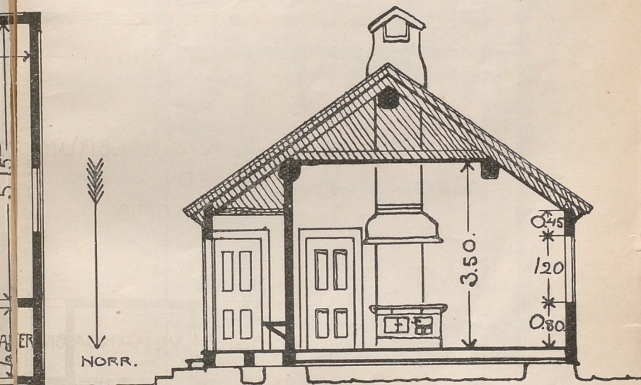
SEKSION I A.—B.
