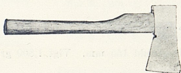
N:o 20. Köksyxa med skaft. Helpolerad. Skaftlängd 370 mm. Eggbredd 80 mm. Vigt 900 gr. Pris Kr. 1: 25.
