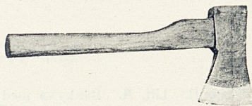
N:o 19. Köksyxa med skaft och skena. Skaftlängd 370 mm. Eggbredd 100 mm. Vigt 1,000 gr. Pris Kr. 1: 25.
