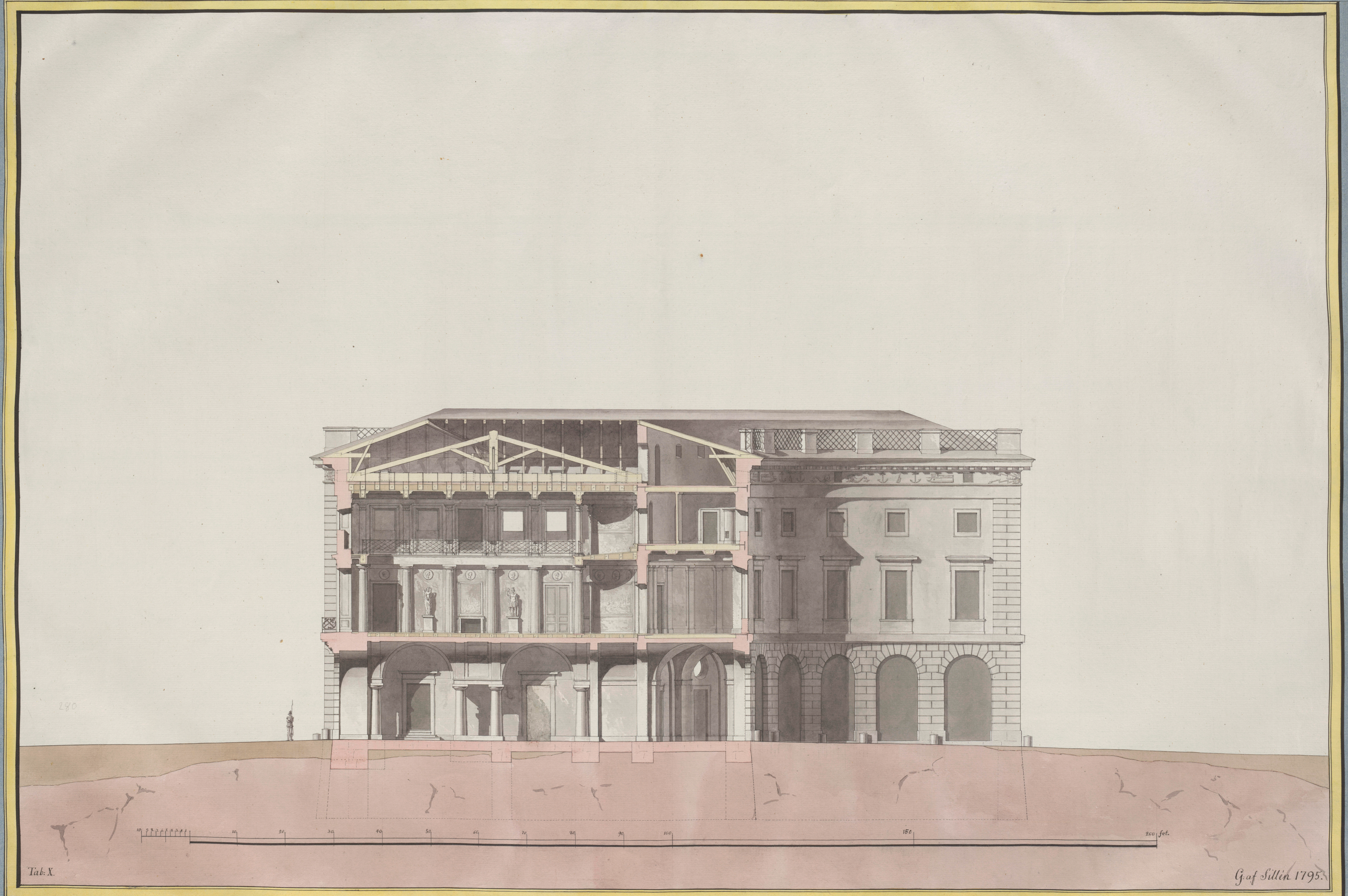
Genomskärning af Samma Bygnad, efter Linien AB.
