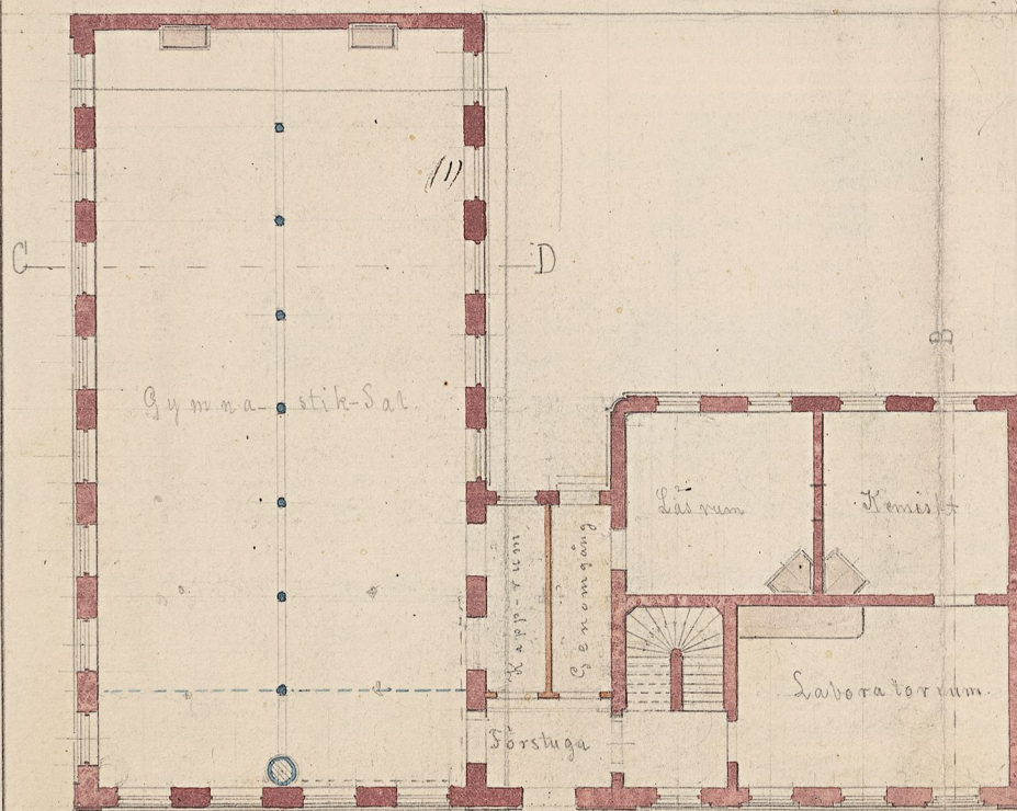
Plan af Bottenvåningen
