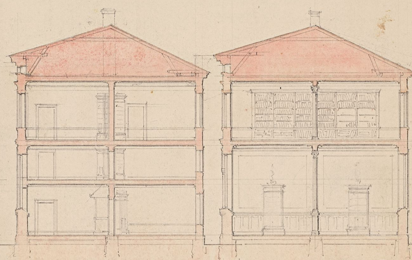
Trägesomskäring vid linier A-B Dito vid C-D
